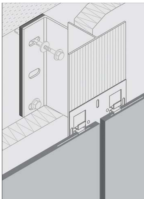
الف- نمونه اجرای اتصال لوبیایی به تیر در اجرای خشک نمای سرامیکی
