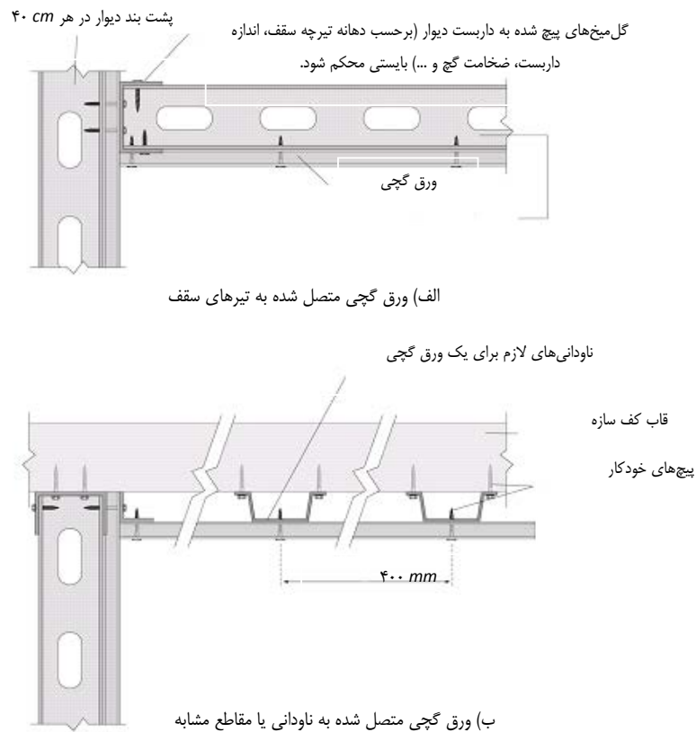
شکل پ۶-۳۳-سقف پانل گچی مستقیم وصل شده به سازه نمونه‌هایی از سقف‌های کاذب نوع الف
