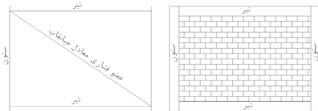
(ب) مدل قاب میانپر
