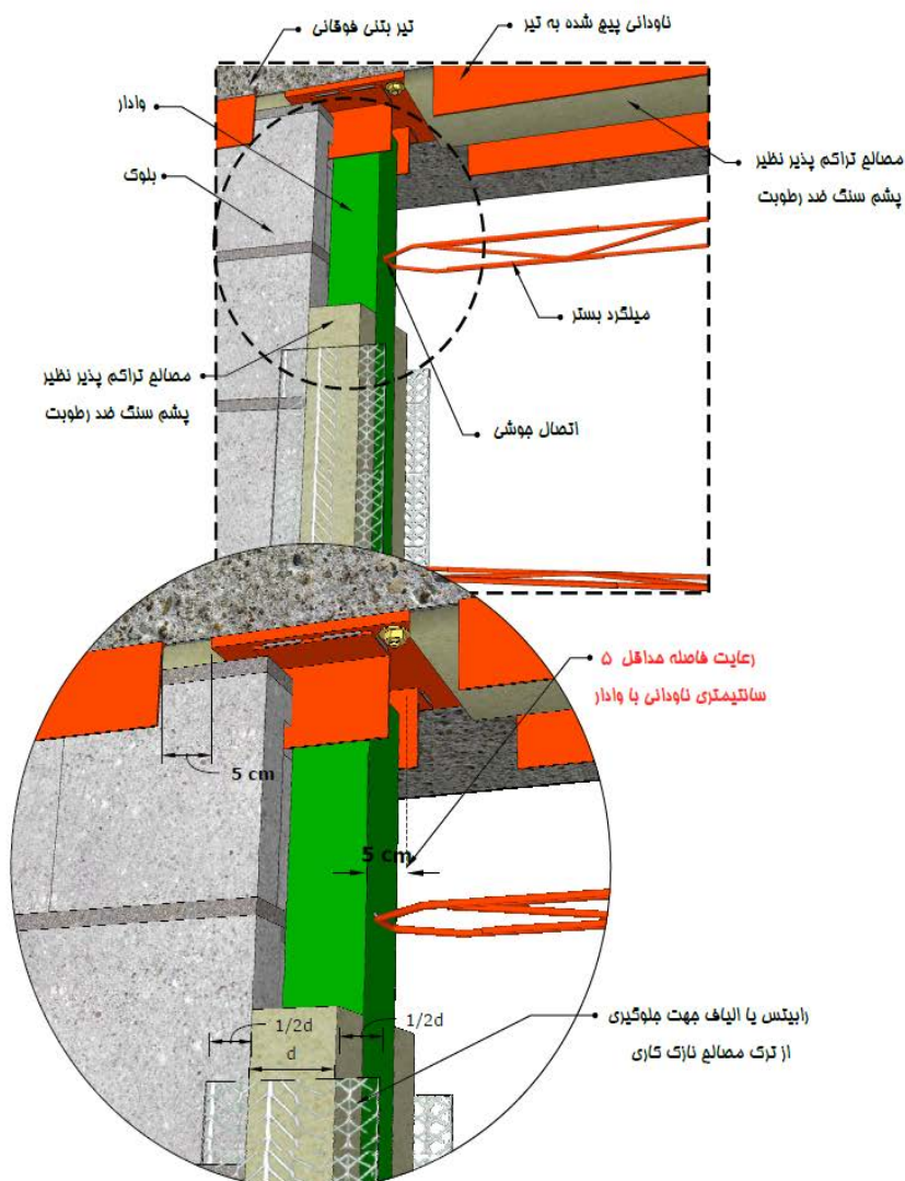
شکل پ ۴-۶- اجرای عایق پشم سنگ و مش الیاف یا رایبتس بر روی وادار
