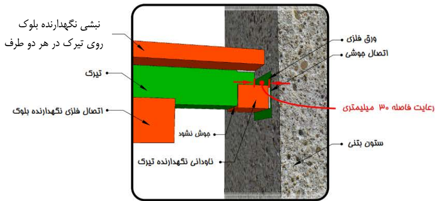
مزییات اتصال تیرک به ستون بتنی
