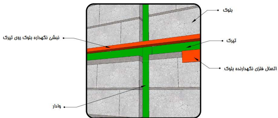
مزییات اتصال تیرک به وادر
