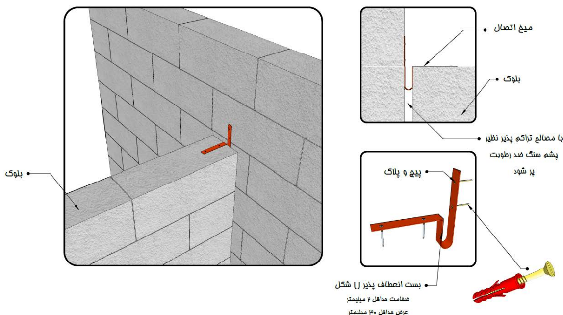
شکل پ-۱۴-۶- اجرای دیوار متقاطع با استفاده از بست انعطاف پذیر
