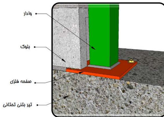
مزییات اتصال وادار میانی روی تیر تمثالی
