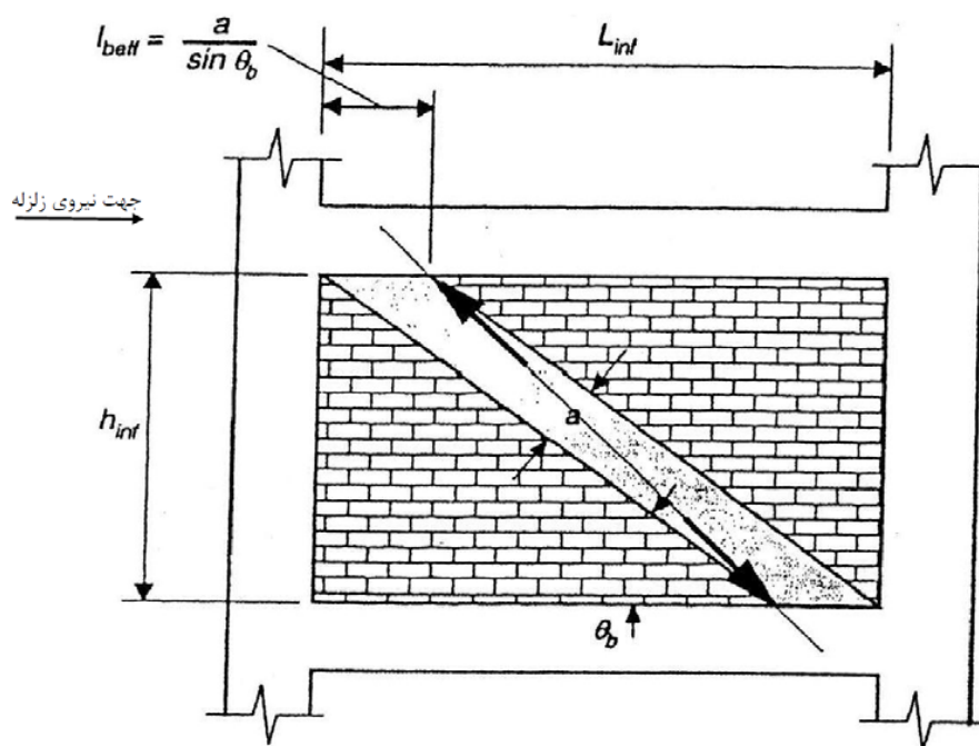
شکل پ۶-۴۳- نیروی وارد به تیر از طرف میانقاب
