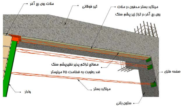
ب- عدم اتصال به سقف و اجرای امان مسلح کننده در رج آخر دیوار شکل پ ۶-۱۱- جزئیات اجرایی در محل تلاقی دیوار با سقف
