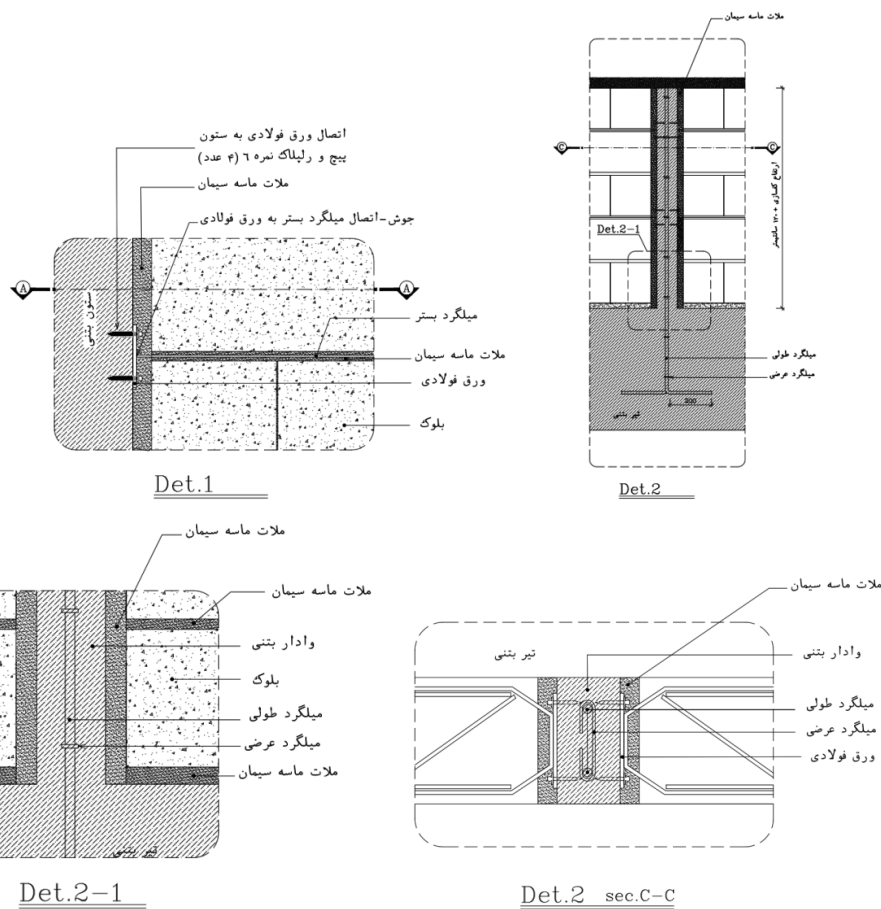
شکل پ-۳۷-۶ جزئیات اجرایی اتصال جان پناه با وادر بتنی
