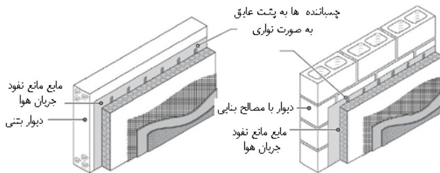
شکل پ-۲۶-۶- نحوه صحیح اجرای نمای سیمانی مسلح شده به مش الیاف و عایق حرارتی بر روی دیوار
