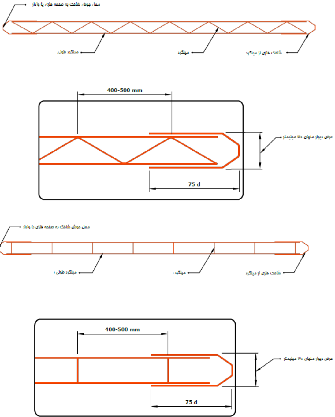
شکل پ ۶-۲- میلگرد بستر خرابایی یا نرده‌بانی
