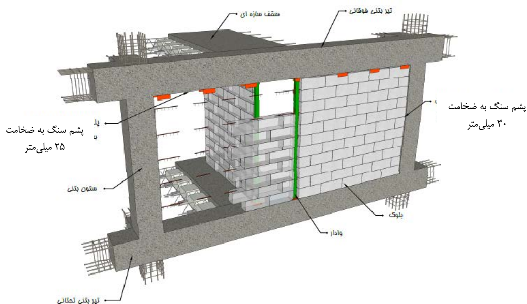
الف- نمای سه بعدی اجرای دیوارهای متقاطع
