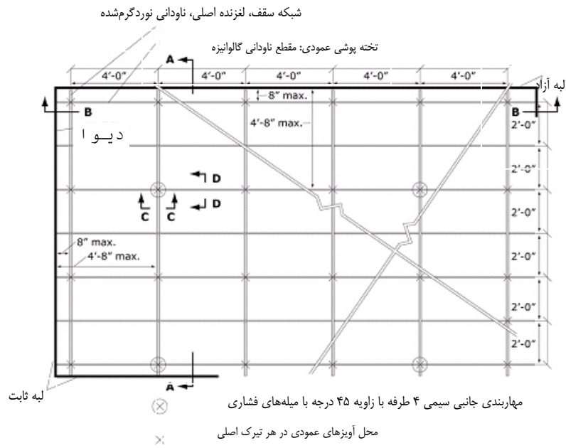
شکل پ ۳۳-۶- پلان مهاربندی عرضی برای شبکه سقف سنگین معلقی (جزئیات مقاطع در شکل پ ۲۹-۶ ارائه شده است)
