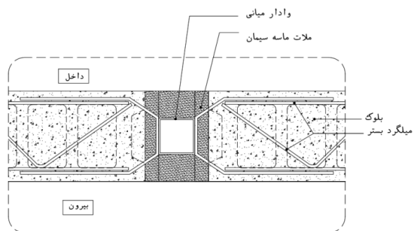
Det.3 sec.A-A
