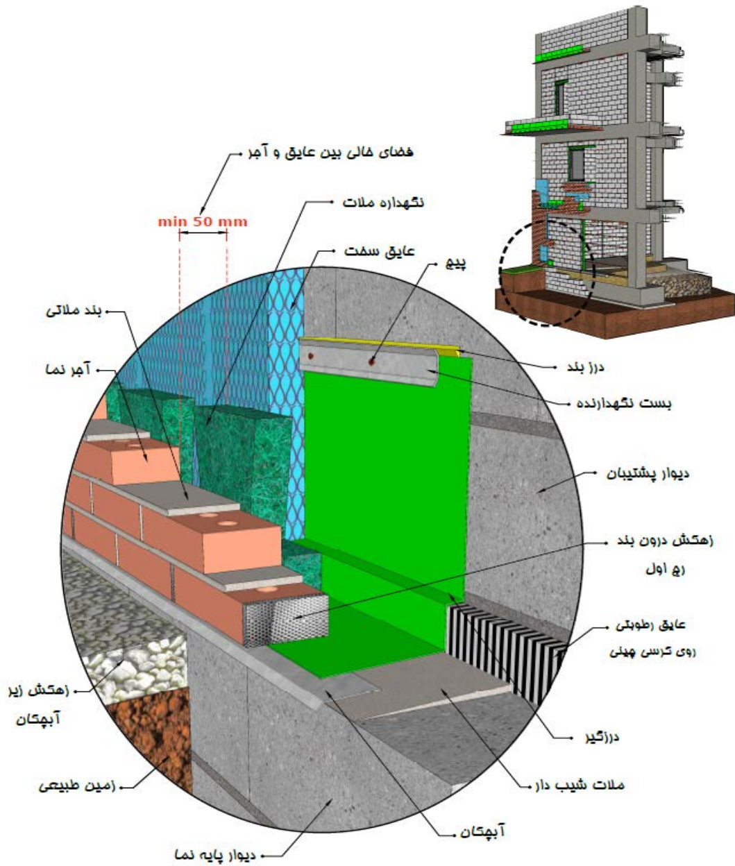
شکل پ ۶-۲۹-جزییات اجرای نمای آجری
