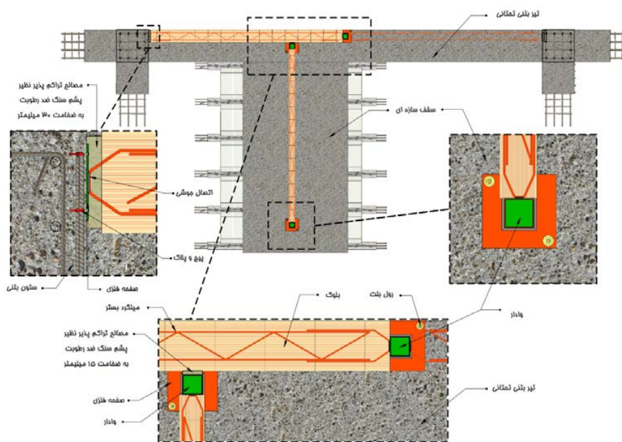
ب- اجرای دیوار متقاطع از پلان
