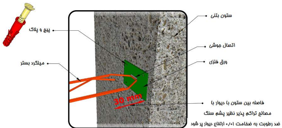
مزییات اتصال میگردد بستر به ستون بتنی
